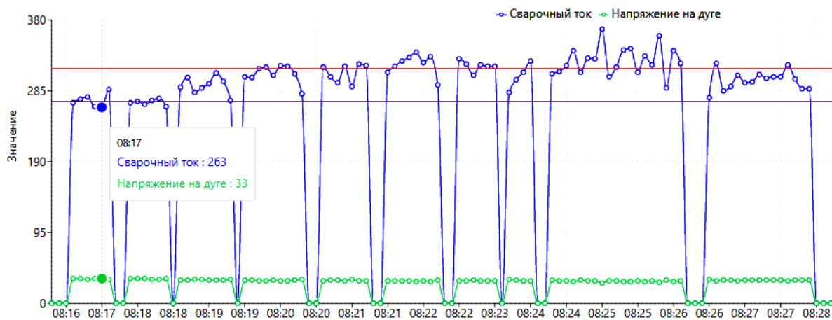
Рис. 2. Результаты мониторинга сварочных процессов
