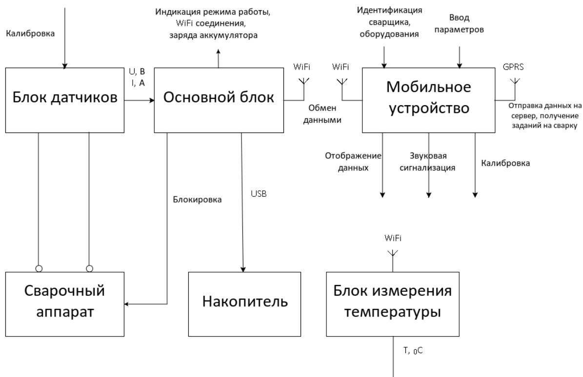
Рис. 1. Структурная схема программно-аппаратного комплекса
