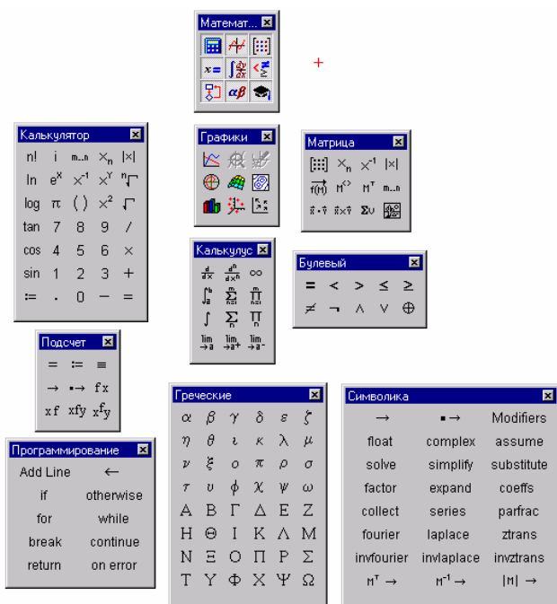
Рис. 3. Панель инструментов Математика с раскрытыми палитрами
