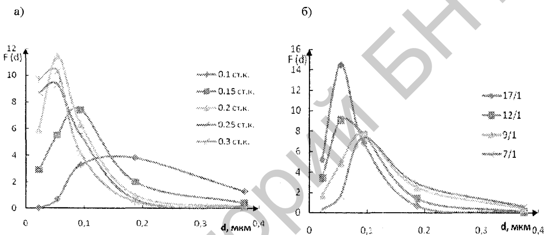
Рис. 3. Гранулометрический состав композиционных порошков, полученных механическим легированием шихты Fe-Al-C_{17}H_{35}COOH при различных значениях заполнения рабочей камеры шарами (а) и соотношении объемов рабочих тел и шихты (б)
