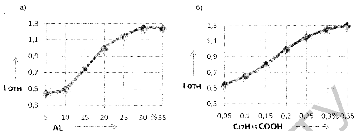
Рис. 5. Влияние содержания в исходной шихте алюминия (а) и стеариновой кислоты (б) на относительную износостойкость покрытий: а – содержание 0,20 % C_{17}H_{35}COOH ; б – содержание 20 % Al
