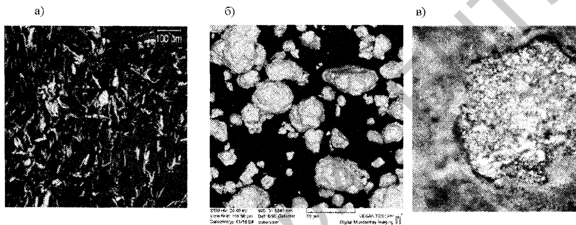
Рис. 2. Форма, размер и структура частиц порошковой композиции Fe-Al-C 17 H 35 COOH, подвергнутой обработке в механореакторе. Продолжительность обработки: а – 2 ч; б – в – 8 ч
