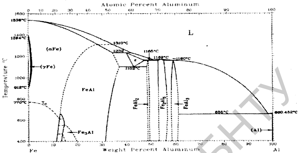
Рис. 1. Диаграмма состояния Fe-Al [10]
