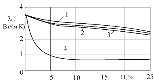
Рис. 3. Расчетные зависимости теплопроводности от пористости отложений с учетом парогазовой пористости: 1 – Ландау – Лифшиц; 2 – Бир; 3 – Лорентц – Лорентц; 4 – Цвиклер
