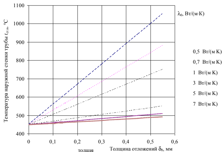
Рис. 2. — — — — — зависимость температуры стенки трубы от толщины отложений; — — — — — 0,5 Вт/(м·К); — — — — — 0,7; — — — — — 1; — — — — — 3; — — — — — 5; — — — — — 7,0 Вт/(м·К)
