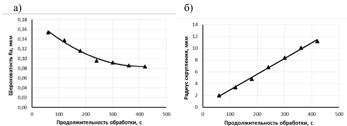
Рис. 1. Влияние продолжительности обработки на изменение шероховатости поверхности образцов (а) и на изменение радиуса скругления (б)
