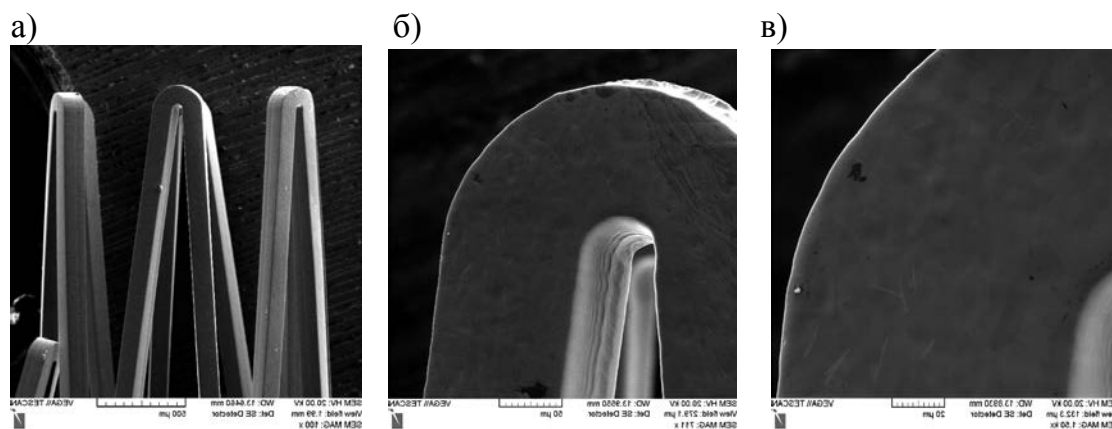
Рис. 2. SEM фотографии поверхности стента: а – увеличение x100; б – увеличение x700; в – увеличение x1500
