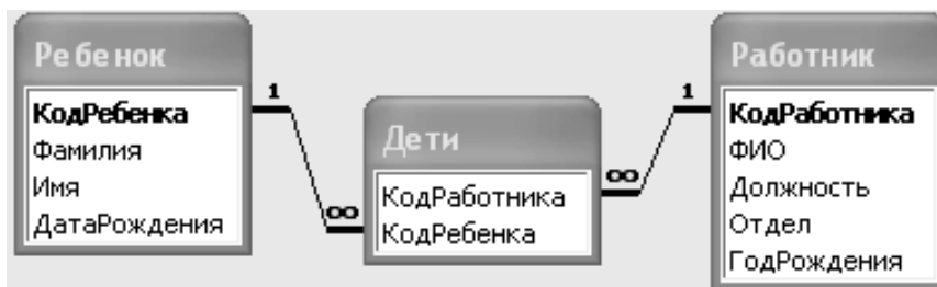
Рис. 7.10. Схема базы данных «Дети»
