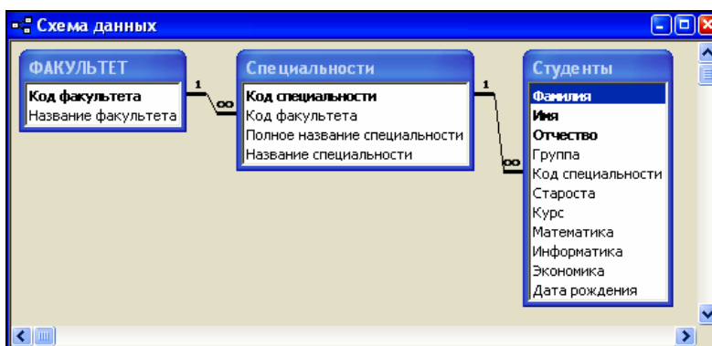
Рис. 1.6. Пример схемы данных
