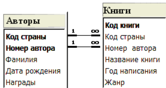
Рис. 7.3. Схема базы данных «Книги»
