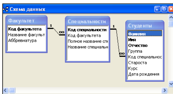
Рис. 2.3. Схема данных базы данных «Студенты»
