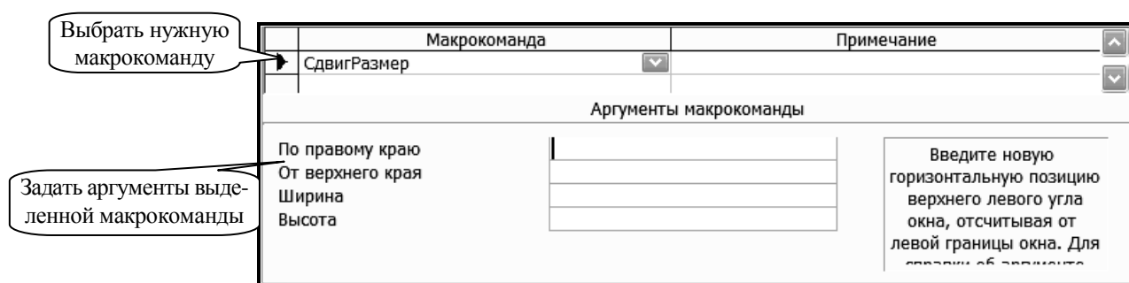
Рис. 10.1. Конструирование макроса
