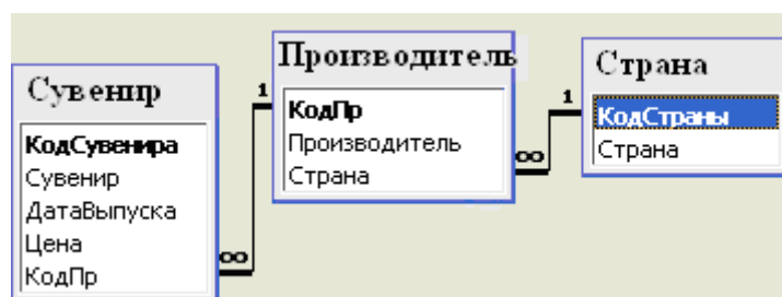
Рис. 7.6. Схема базы данных «Сувениры»
