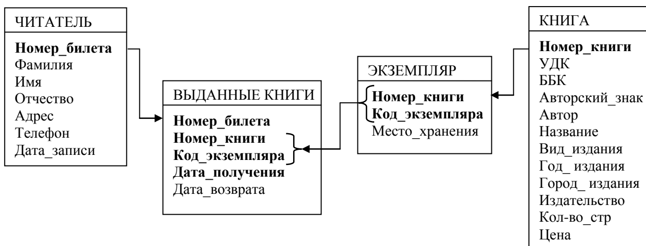
Рис. 12.4. Информационно-логическая модель (ИЛМ) базы данных «Библиотека»
