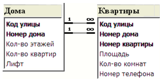
Рис. 7.4. Схема базы данных «Дома»
