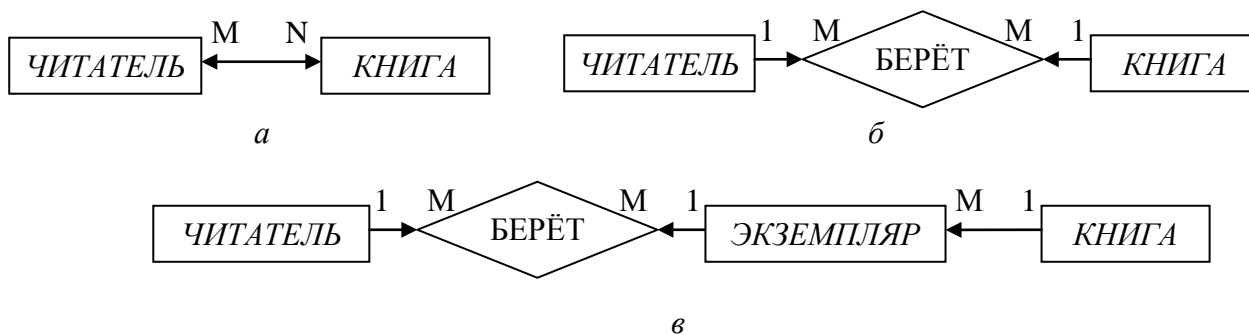
Рис. 12.3. Построение ER-диаграммы
