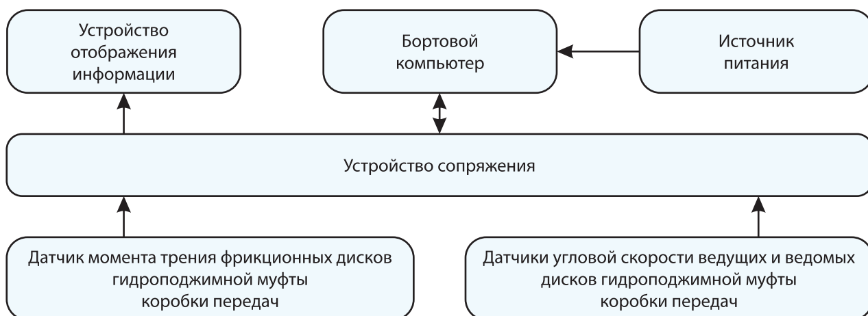
Структурная схема системы бортового диагностирования степени износа фрикционных дисков гидроподжимных муфт коробки передач
