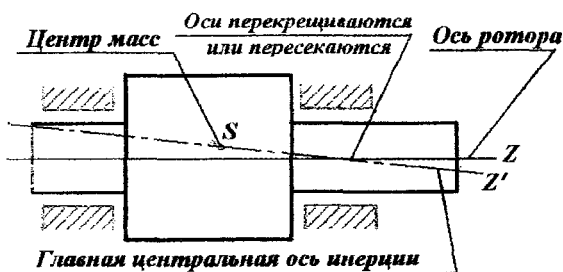
Рис. 4. Динамическая неуравновешенность ротора
