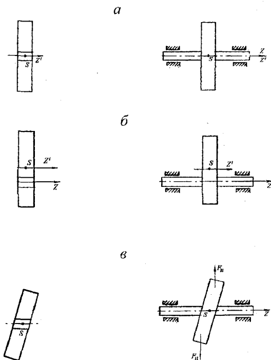
Рис. 5. Появление неуравновешенности ротора за счет нарушений технологии изготовления и сборки
