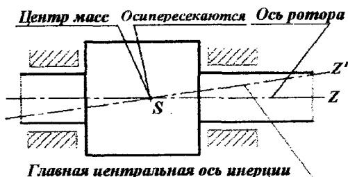
Рис. 3. Моментная неуравновешенность ротора
