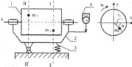
1 – ротор, 2 – рама, 3 – пружина, 4 – индикатор; I и II – плоскости уравновешивания.
