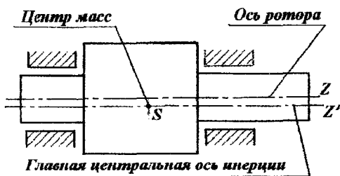
Рис. 2. Статическая неуравновешенность
