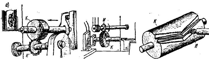
Циклограмма
