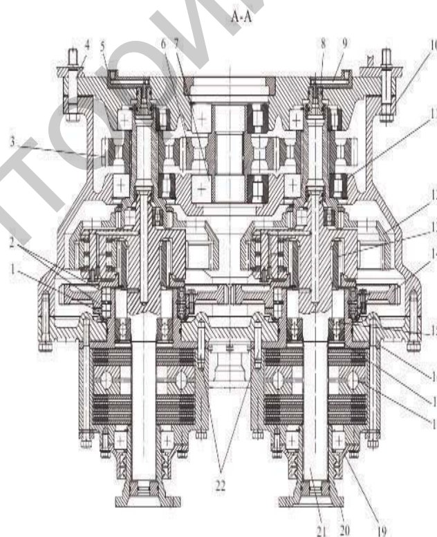
Рисунок 7 - Механизм поворота (продольный горизонтальный разрез)
