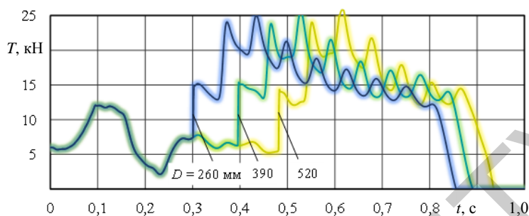
Рис. 11. Зависимость тяжения от удлинения демпфера
