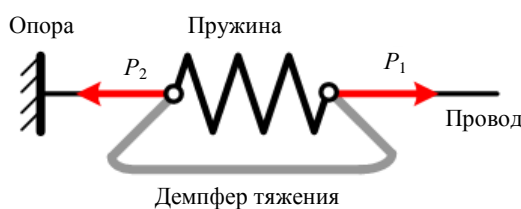
Рис. 2. Расчетная схема для математического моделирования динамики демпфера ( P_1, P_2 – силы, действующие на демпфер тяжения)
