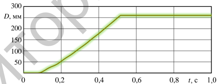
Рис. 9. Удлинение демпфера при коротком замыкании
