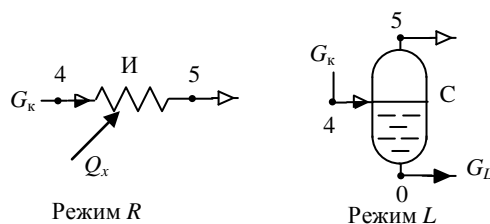
Рис. 3. Схемы ступеней использования охлаждения для различных режимов работы установки: И – испаритель; С – сборник жидкости
