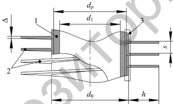
Рис. 1. Элемент незагрязненной биметаллической ребристой трубы: 1 – несущая труба; 2 – ленточное оребрение; 3 – оболочка
