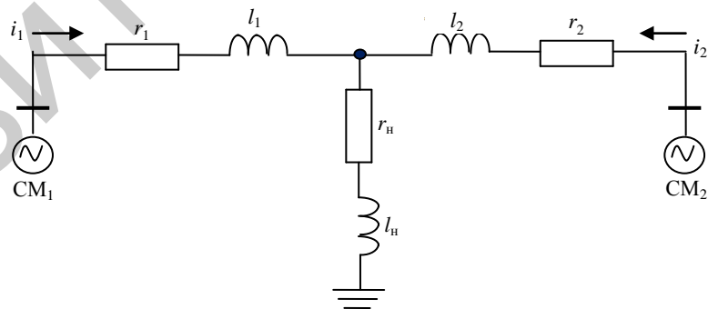
Рис. 1. Синхронная двухмашинная система: CM_1 , CM_2 – синхронная машина; i_1 ( i_{1a} , i_{1b} , i_{1c} ), i_2 ( i_{2a} , i_{2b} , i_{2c} ) – трехфазный ток статора синхронной машины; r_1 , l_1 ( r_2 , l_2 ) – активное сопротивление и индуктивность линии; r_n , l_n – активное сопротивление и индуктивность нагрузки
