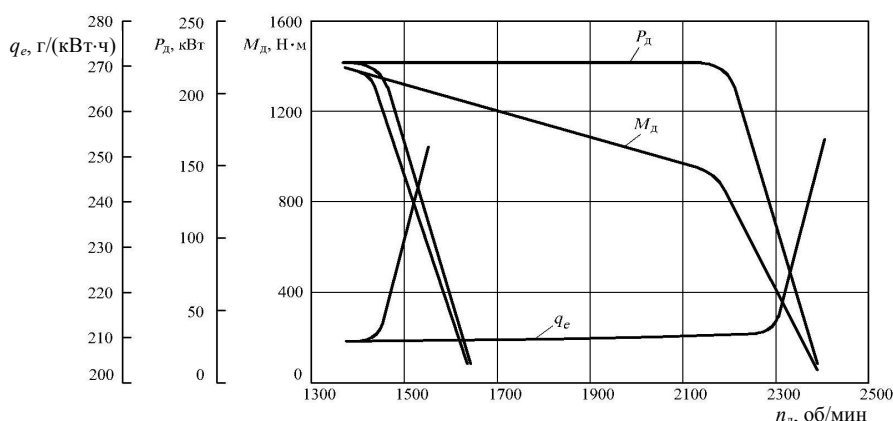
Рис. 1. Типовая характеристика двигателя фирмы Detroit Diesel серии 40E-8,7LTA мощностью 220 кВт (300 л. с.)
