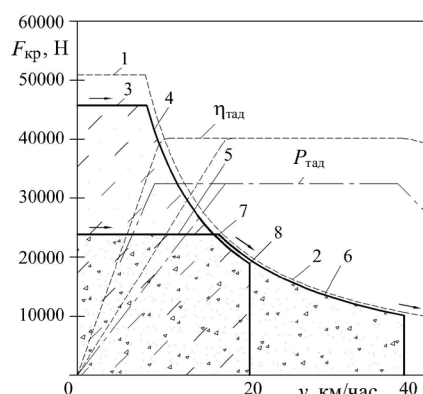
Рис. 5. Потенциальная тяговая характеристика трактора с тяговым электродвигателем
