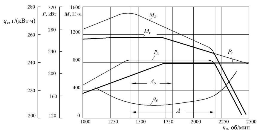
Рис. 3. График совместной работы двигателя внутреннего сгорания и генератора
