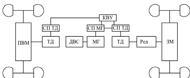
Рис. 7. Структурная схема трактора с приводом каждого моста отдельным электродвигателем (обозначения – на рис. 5)
