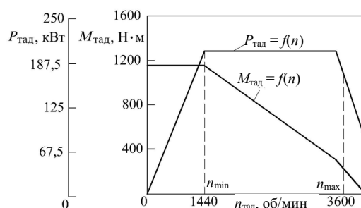
Рис. 6. Характеристика тягового электродвигателя
