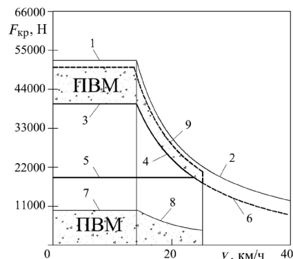
Рис. 8. Потенциальная тяговая характеристика трактора с двумя тяговыми электродвигателями
