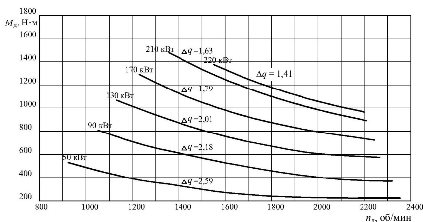
Рис. 2. Характеристики двигателя Detroit Diesel серии 40E-8,7LTA мощностью 220 кВт (300 л. с.) при фиксированных мощностях
