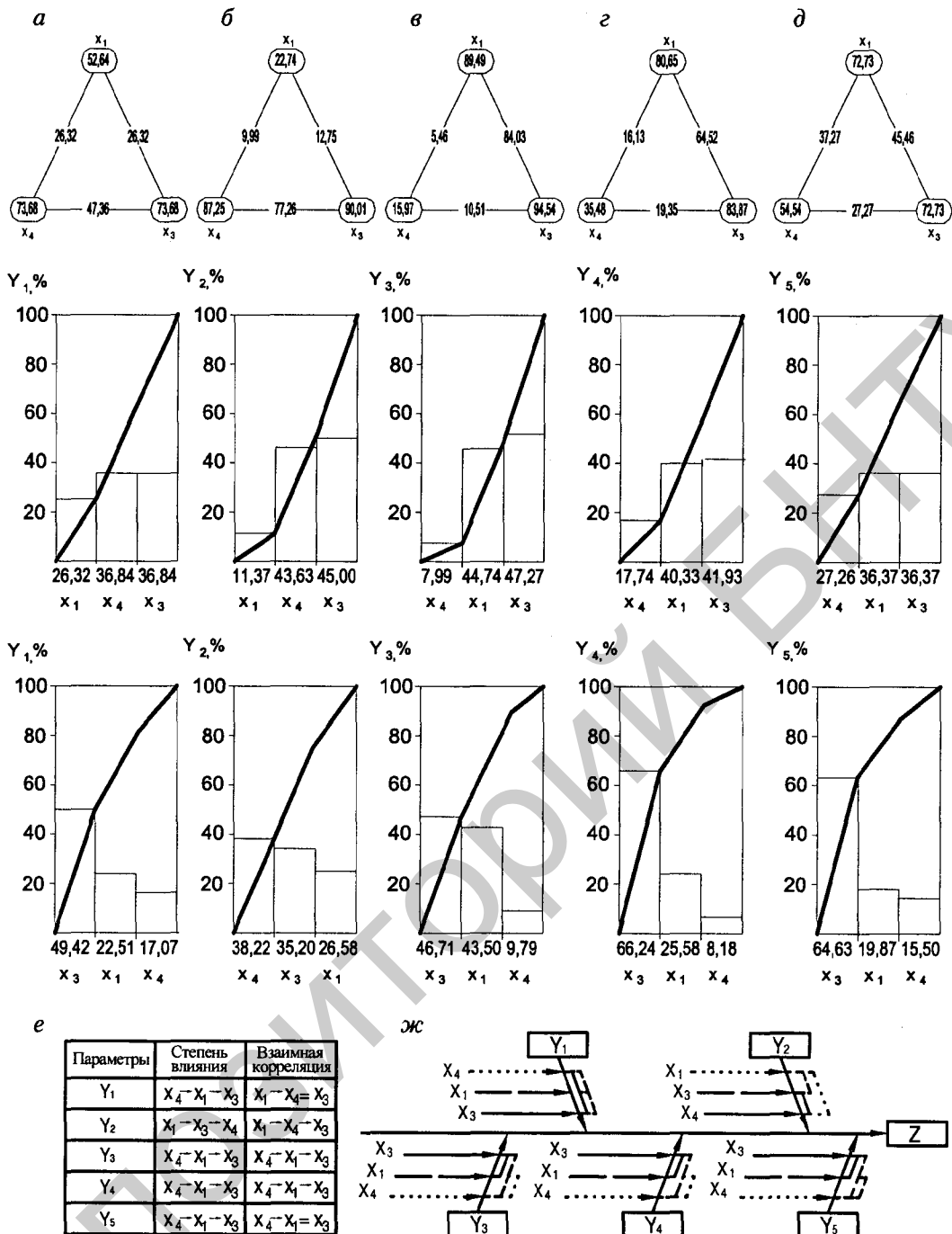
Рис. 2. Управление специальным процессом комбинированной упрочняюще-размерной термомеханической обработки износостойкого покрытия порошком ПГ-10Н-01 по комплексу параметров: HRC (а), U_H (б), Sm_w (в), Ra (г), K (д), с учетом влияния и взаимосвязи факторов (е) на диаграмме «причины—результат» (ж)
