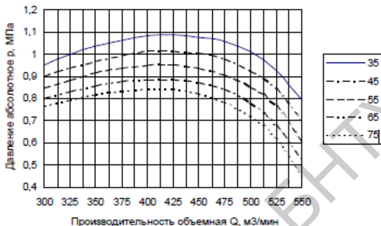
Рисунок 1 – Зависимость характеристик турбокомпрессора K500-61-5 температуры воздуха после промежуточных воздухоохладителей
