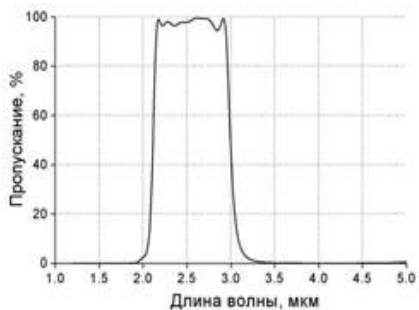
Рисунок 5 – Полосовой пропускающий фильтр
