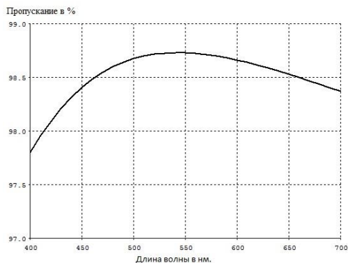
Рисунок 1 – Однослойное просветляющее покрытие
