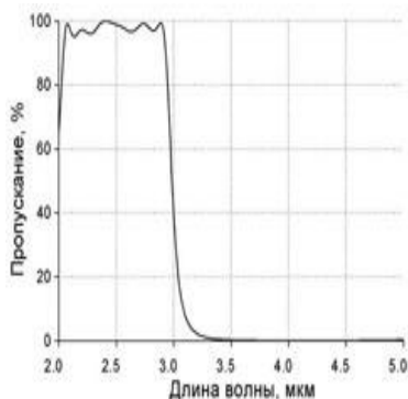
Рисунок 4 – Отрезающий коротковолновый фильтр
