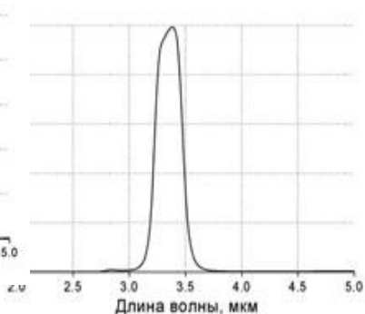
Рисунок 6 – Узкополосной пропускающий фильтр
