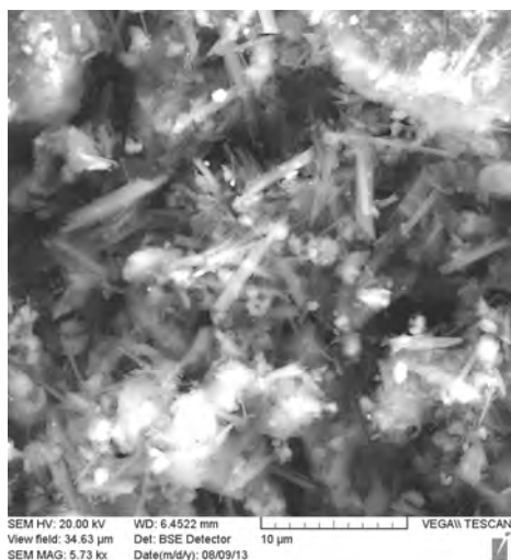
Рис. 2. Шлак, затворенный сульфатным активатором
