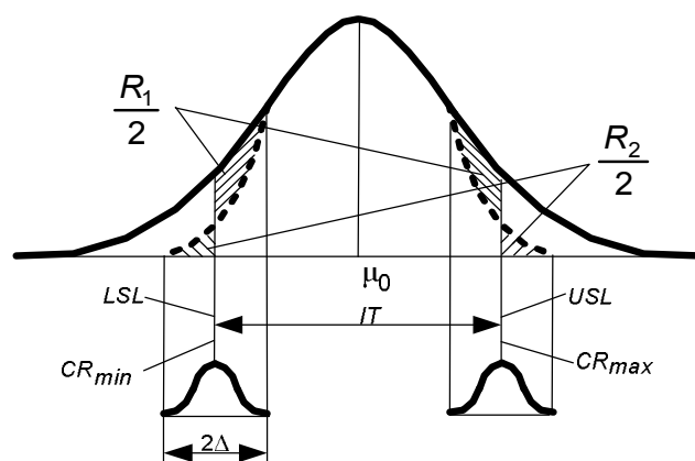
Рисунок 1 – Графическая интерпретация метрологической модели операционного контроля применительно к контролю продукции: USL, LSL – предельные значения контролируемого параметра (верхнее и нижнее соответственно); IT – допуск контролируемого параметра; CR_{min}, CR_{max} – приемочные границы; \mu_0 – математическое ожидание контролируемого параметра; R_1 – риск первого рода; R_2 – риск второго рода; \Delta – погрешность измерения
