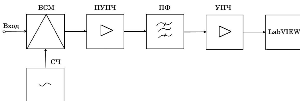
Рисунок 1 – Структурная схема измерительного комплекса
