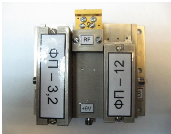
Рисунок 3 – Внешний вид преобразователя частоты
