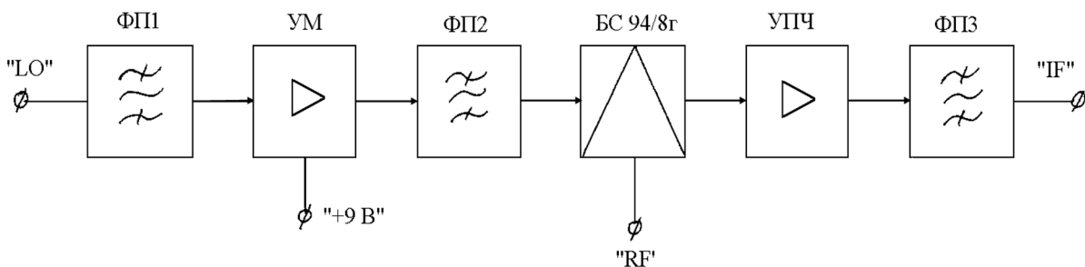
Рисунок 2 – Структурная схема преобразователя частоты на восьмой гармонике
