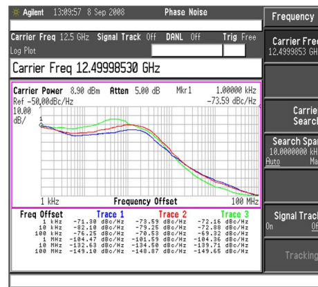
Рисунок 7 – Фазовые шумы синтезатора частоты с целочисленным коэффициентом деления
