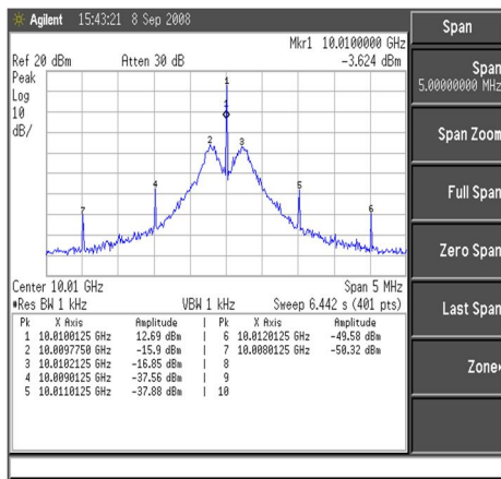
Рисунок 6 – Спектр выходного сигнала синтезатора частот при частотной манипуляции
