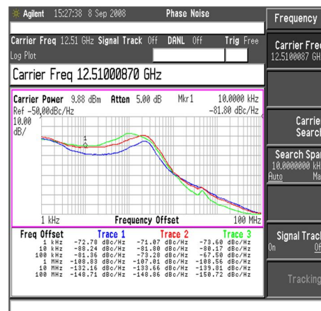
Рисунок 8 – Фазовые шумы синтезатора частоты с дробным коэффициентом деления
