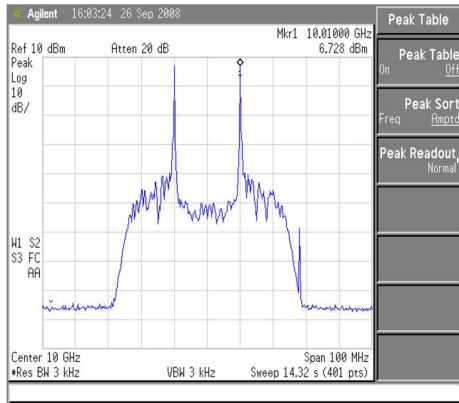
Рисунок 5 – Спектр сигнала синтезатора частот при частотной манипуляции
