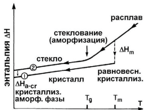
Рисунок 4 – Схема изменения энтальпии при получении АС закалкой расплава и при кристаллизации аморфной фазы в условиях нагрева до температур ниже T_g (по материалам [10])
