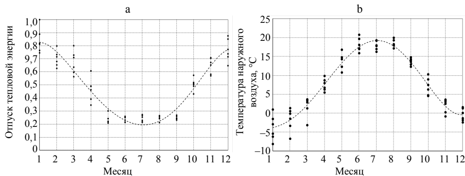
Рис. 3. Отпуск тепловой энергии районной котельной (а) на фоне динамики изменения температуры наружного воздуха (b) в период 2015–2020 гг.
