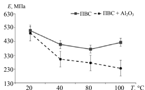
Рис. 6. Термомеханические свойства однослойных полимерных покрытий на основе поливинилового спирта Fig. 6. Thermomechanical properties of single-layer PVA based coatings
