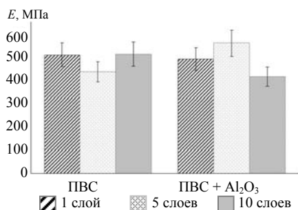
Рис. 4. Значения модуля упругости для пленок на основе поливинилового спирта Fig. 4. Values of the elastic modulus for the PVA based films
