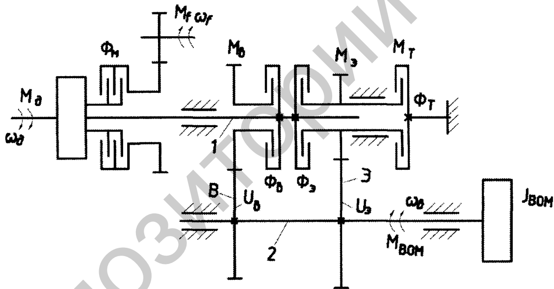
Рис. 1. Двухмассовая динамическая модель системы с элементами узлов ВОМ: 1, 2 – ведущий и ведомый ВОМ; \Phi_n и \Phi_3 – фрикционы высшей и экономичной передач; M_d и \omega_d – крутящий момент и угловая скорость вала двигателя, приведенные к валу включаемой ФМ; I_d – момент инерции движущихся частей двигателя и связанных с ними деталей, приведенный к валу включаемой ФМ; M_{\text{ВОМ}} и I_{\text{ВОМ}} – момент сопротивления движению и момент инерции ВОМ тракторного агрегата; \omega_n – угловая скорость ведомого вала; u_n и u_3 – передаточные числа; \Phi_n – фрикционная передача главной муфты сцепления; M_f – момент сопротивления перекачиванию и угловая скорость при перекачивании трактора
