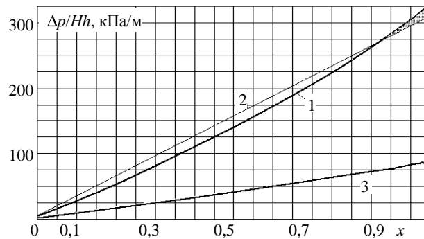
Рис. 2. Зависимость перепада давления от паросодержания: 1, 2 – (\rho_w)_f = 22 \text{ кг}/(\text{м}^2 \cdot \text{с}) ; 3 – 11; p = 3,0 \text{ МПа} ; d = 2 \text{ мм} ; \varepsilon = 0,37 , «вода + пар», расчет по [9]
