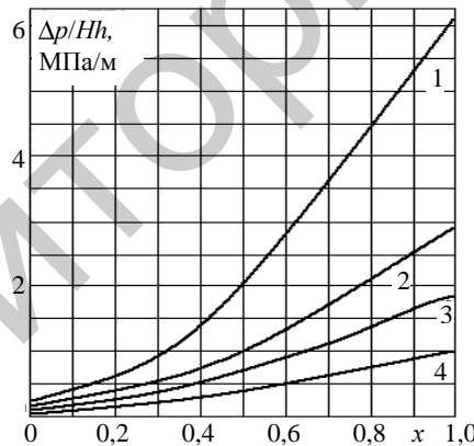
Рис. 1. Зависимость перепада давления от паросодержания: 1 – (\rho w)_f = 55 \text{ кг}/(\text{м}^2 \cdot \text{с}) , абсолютное давление p = 0,9 \text{ МПа} ; 2 – 55, 2,0; 3 – 55, 3,0; 4 – 22, 0,9; диаметр микровзла d = 2 \text{ мм} ; пористость \varepsilon = 0,37 , «вода + пар», расчет по [9]
