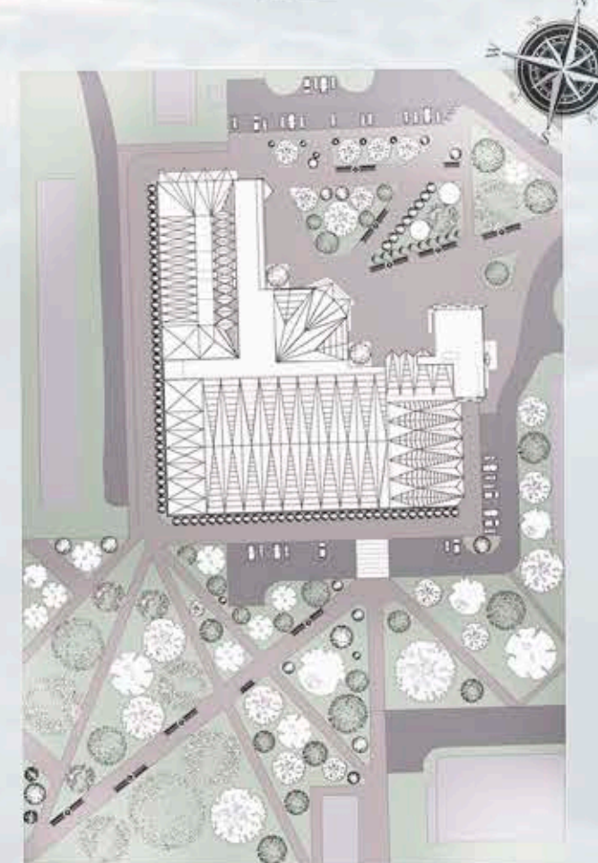
Генеральный план 1:500
